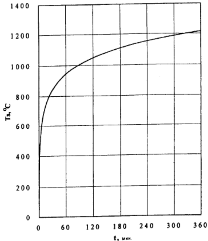
Рисунок 1 - Стандартный температурный режим
