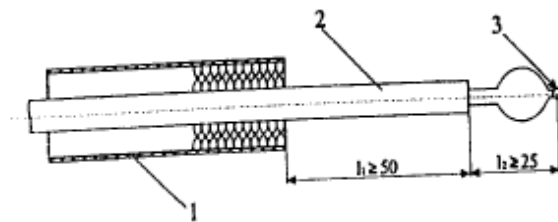
1-теплозащитная оболочка; 2-защитный кожух; 3-измерительный спай Рисунок Б.1 - Термопара для измерения температуры в печи
