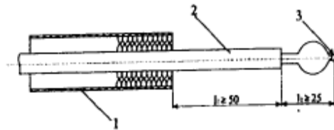
1 - теплозахисна оболонка; 2 - захисний кожух; 3 - вимірювальний спай Рисунок Б. 1 - Термопара для вимірювання температури в печі
