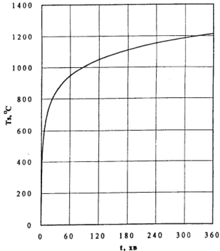
Рисунок 1 - Стандартний температурний режим
