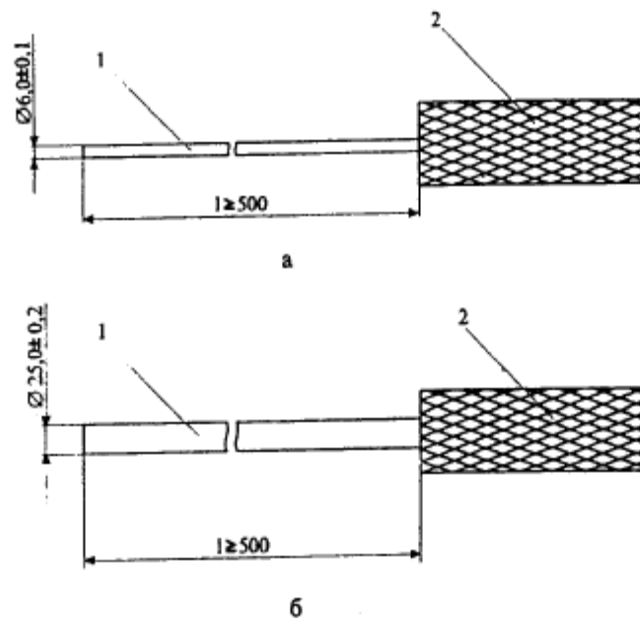
1 - цилиндрический стальной стержень; 2 - держатель Рисунок Б.3 - Щупы для оценки целостности диаметром 6 мм (а) и диаметром 25 мм (б)
