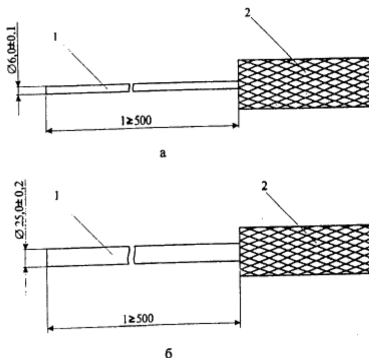
Рисунок Б.3 - Щупи для оцінки цілісності діаметром 6 мм (а) та діаметром 25 мм (б)
