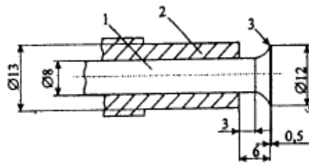
1-защитный кожух; 2-теплозащитная оболочка; 3-медный диск Рисунок 5.2 - Переносная термопара
