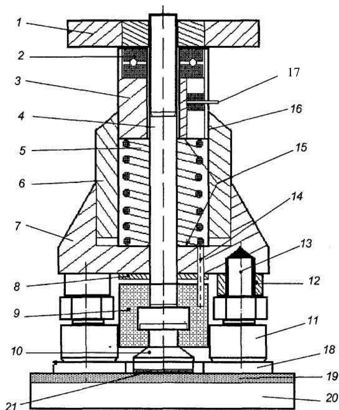
Адгезиметр
