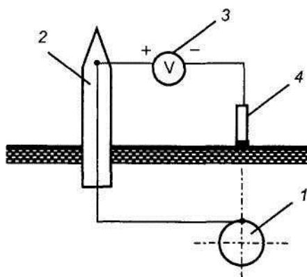
1 – трубопровід; 2 – пункт вимірювання; 3 – вольтметр; 4 – мідносульфатний електрод, що розташовують над визначеною віссю труби.
