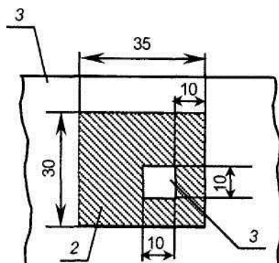
Рисунок Е.1 – Пристрій СМ-1 для випробування захисних покриттів на основі мастикових матеріалів
