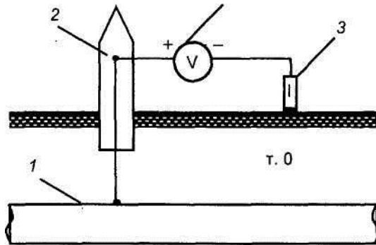
1– трубопровід; 2– пункт вимірювання; 3– перший мідносльфатний електрод, що розташовують над визначеною віссю труби; 4– вольтметр.
