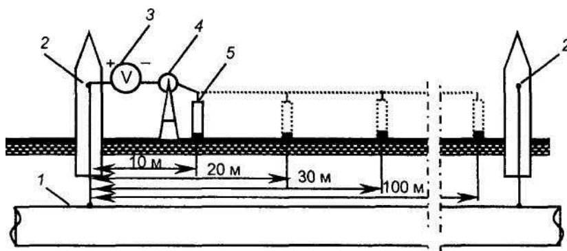
1 – трубопровід; 2 – пункт вимірювання; 3 – вольтметр; 4 – котушка з проводом; 5 – мідно сульфатний електрод.
