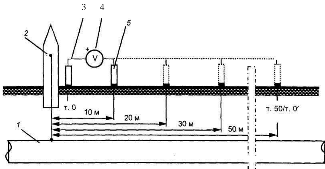
1 – трубопровід; 2 – пункт вимірювання; 3 – нерухомий мідносльфатний електрод, відносно якого вимірюють потенціал першого переносного електрода; 4 – вольтметр; 5 – перший рухомий мідносльфатний електрод.
