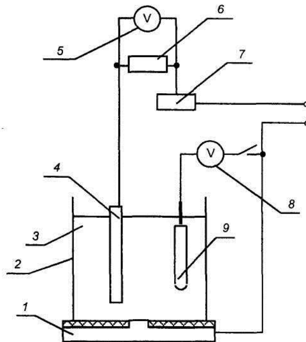
1 – випробовуваний зразок; 2 – труба з поліетилену; 3 – електроліт; 4 – інертний анод; 5 і 8 – вольтметри; 6 – еталонний опір; 7 – реостат; 9 – електрод порівняння.
