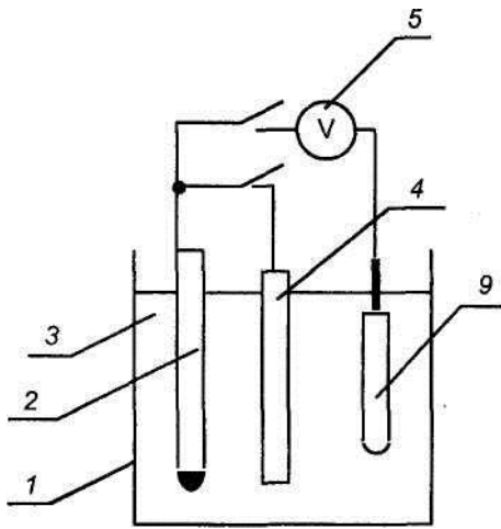
1 – посудина; 2 – випробовуваний зразок; 3 – електроліт; 4 – магнієвий анод; 5 – вольтметр; 9 – електрод порівняння.
