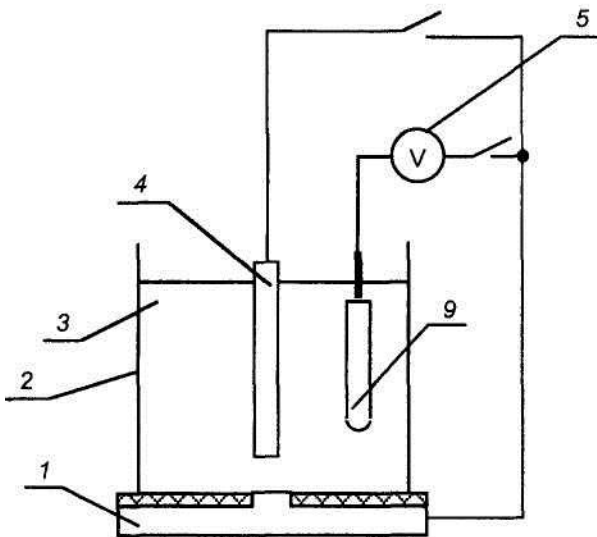
1 – випробовуваний зразок; 2 – труба з поліетилену; 3 – електроліт; 4 – магнієвий анод; 5 – вольтметр; 9 – електрод порівняння.
