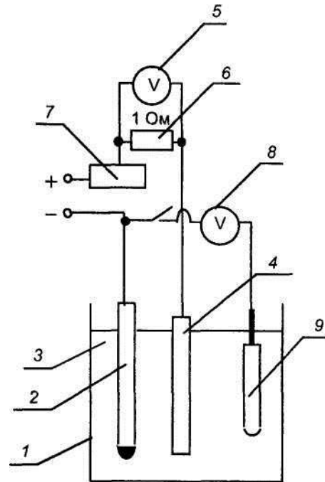
1 – посудина; 2 – випробовуваний зразок; 3 – електроліт; 4 – інертний анод; 5 і 8 – вольтметри; 6 – еталонний опір; 7 – реостат; 9 – електрод порівняння.
