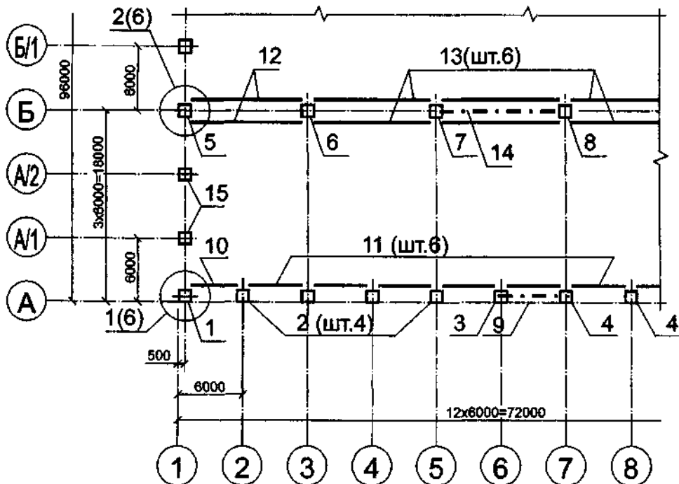
Схема розміщення колон і підкранових балок
