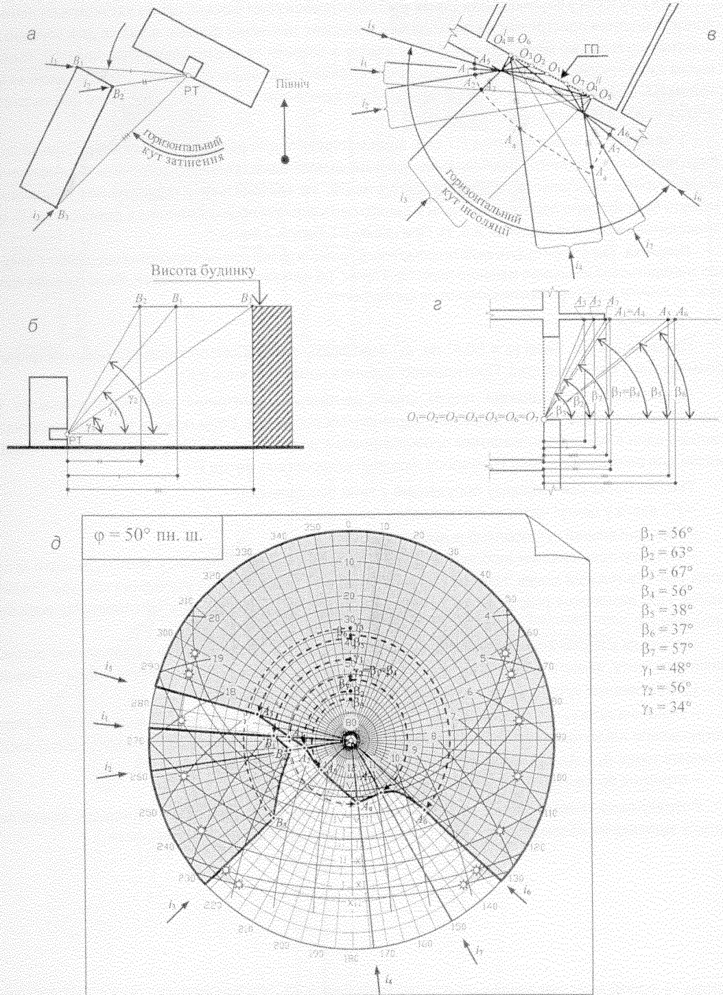
а – визначення горизонтального кута затінення сусіднім будинком та напрямів для побудови тіньової маски за-будови; б – визначення вертикальних кутів затінення сусіднім будинком; в – визначення горизонтального кута інсоляції та напрямів для побудови тіньової маски світлопрорізу; г – визначення вертикальних кутів інсоляції; д – побудова суміщеної тіньової маски
