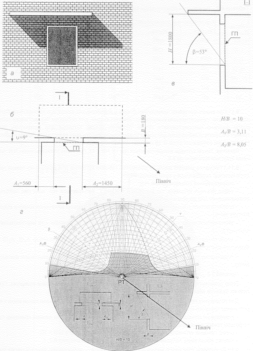
Рисунок 9.7 – Приклад побудови тіньової маски вікна з використанням тіньового кутоміра для розрахунку повної тривалості інсоляції приміщення
