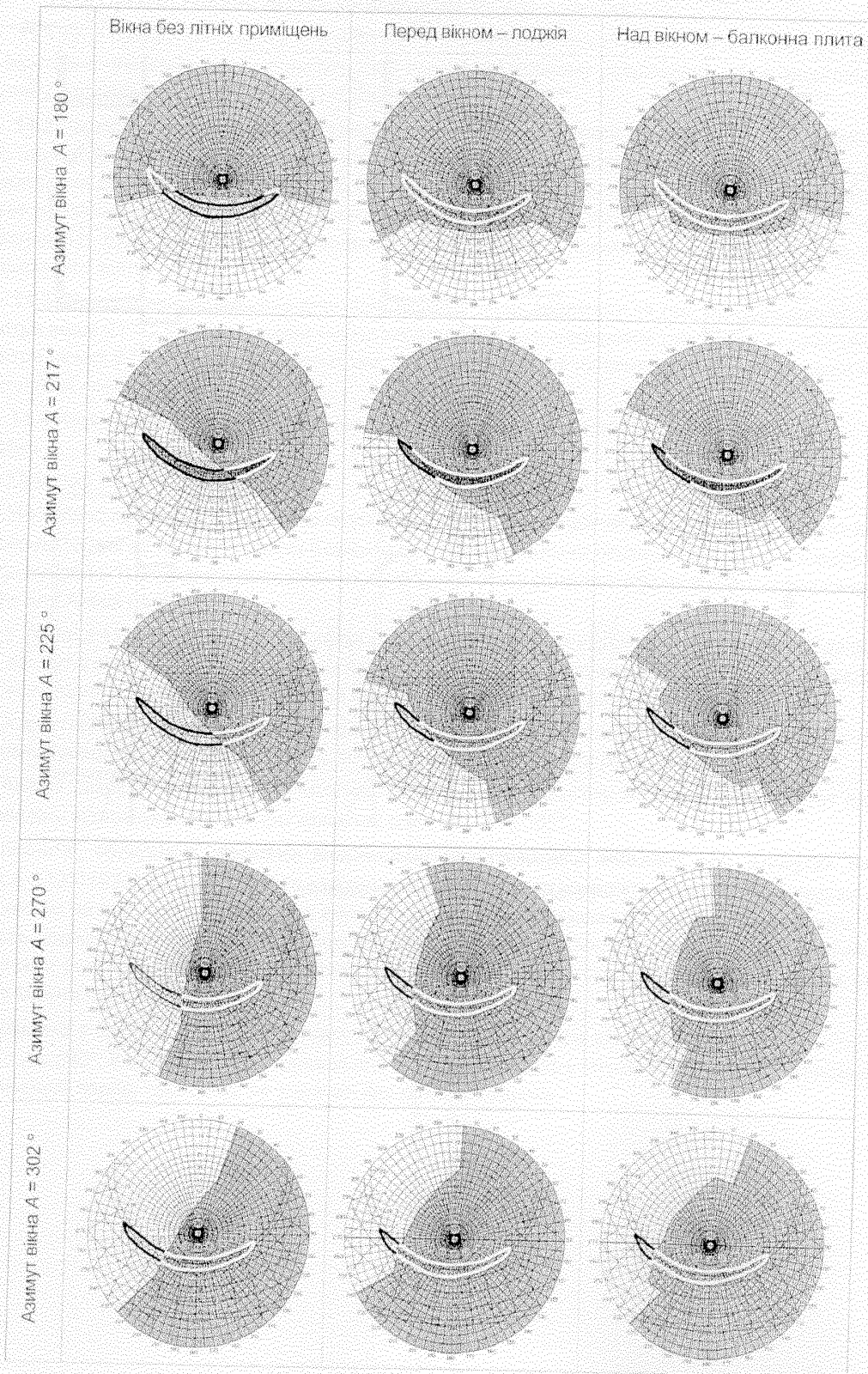
Таблиця 11.1 – Тіньові маски вікон при різній орієнтації
