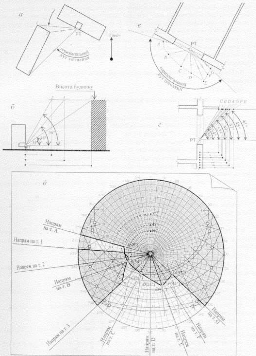
а – визначення горизонтального кута затінення сусіднім будинком та напрямів для побудови тіншової маски за будови; б – визначення вертикальних кутів затінення сусіднім будинком, в – визначення горизонтального кута інсоляції та напрямів для побудови тіншової маски світлопрорізу; г – визначення вертикальних кутів інсоляції; д – побудова тіншової маски для розрахунку тривалості інсоляції приміщення
