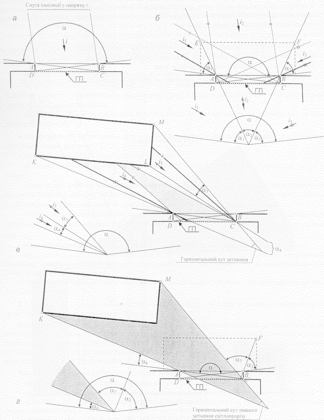
а – світлопроріз без затінення; б – світлопроріз, що затінюється балконною плитою; в – затінення світлопрорізу невисоким будинком; г – затінення світлопрорізу високим будинком
