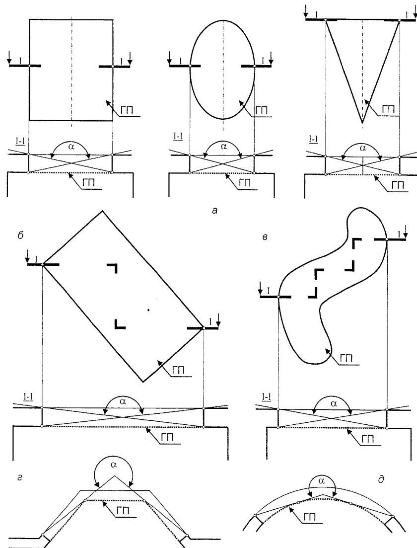
а – у світлопрорізах з вертикальною віссю симетрії; б – у несиметричних світлопрорізах простої форми; в – у світлопрорізах довільної форми; г – у призматичних випуклих світлопрорізах
