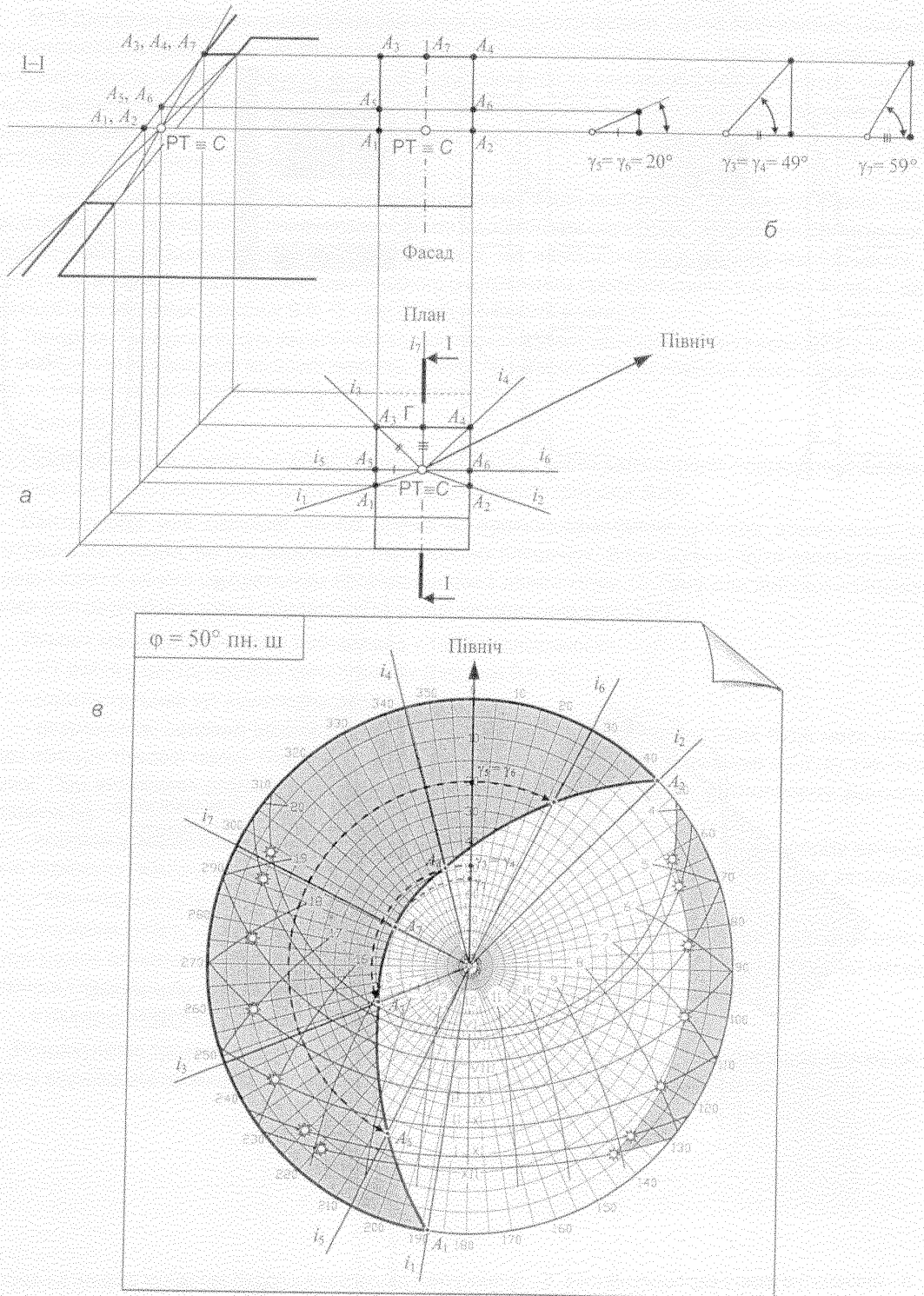
а – задання положення РТ та напрямів для побудови тіньової маски на кресленнях світлопрорізу; б – визначення вертикальних кутів затінення РТ за напрямками; в – побудова тіньової маски
