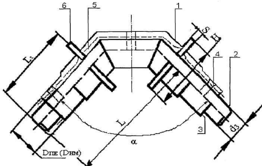
1 - оболонка з поліетилену чи металу, стійкого до впливу атмосферної корозії; 2 - провідна труба зі сталі; 3 - провідники системи сигналізації ушкодження провідної труби та (або) оболонки; 4 - центратори; 5 - ізоляція з пінополіуретану; 6 - нерухома опора; електроізоляційна трубка згідно з ГОСТ 22056 умовно не показана
