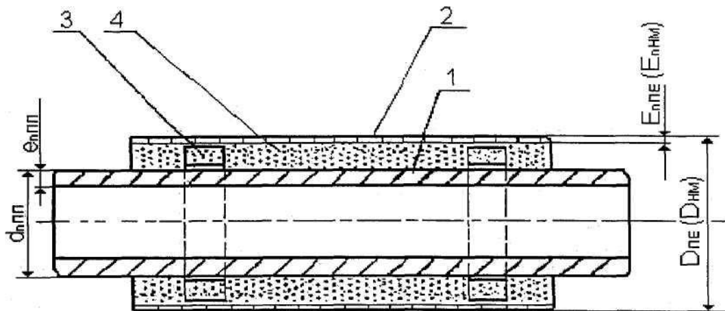
1 - провідна труба з ПП-80тип 3; 2 - оболонка з поліетилену або металу, стійкого до впливу атмосферної корозії; 3 - центратори; 4 - ізоляція
